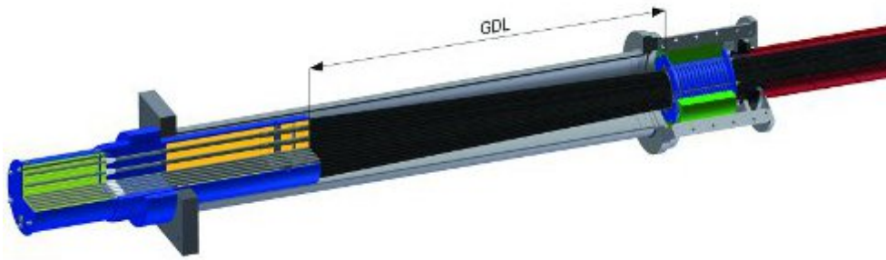
Fot. 1. Warianty zakotwień wantowych z dewiatorem w obudowie
