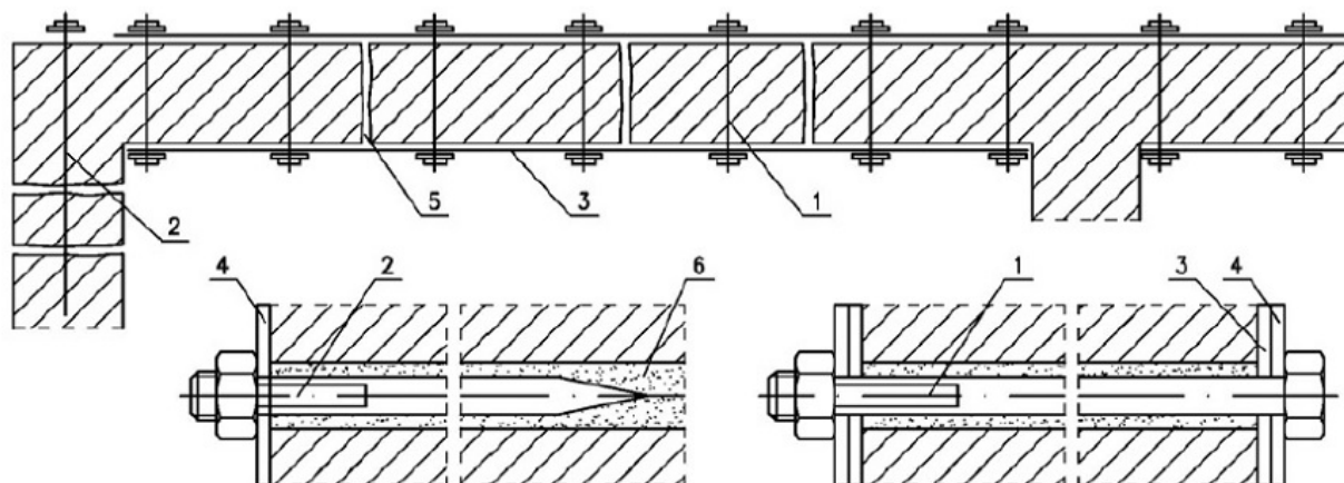
Rys. 4. Wzmocnienie ścian stalowymi płaskownikami i wstępnie sprężonymi sworzniami: 1 - sworzień sprężający, 2 - sworzień wewnętrzny, 3 - płaskowniki stalowe, 4 - podkładki pod sworznie, 5 - pęknięcie w murze wypełnione zaczynem iniekcyjnym, 6 - otwór na sworzień
