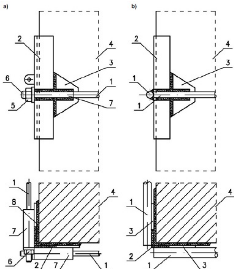
Rys. 6. Szczegóły podpór ściąągów: a)
