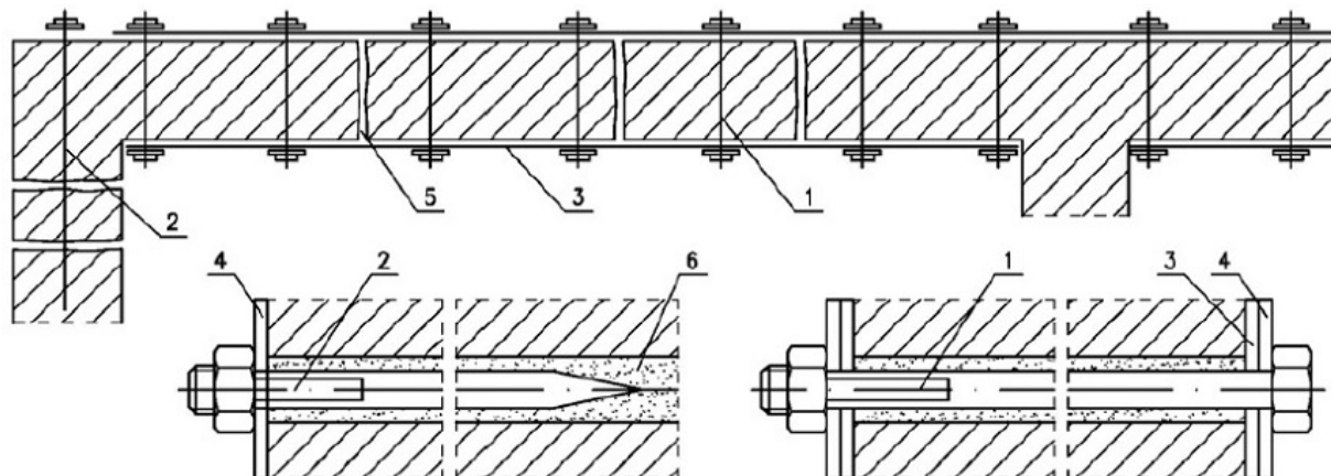
Rys. 4. Wzmocnienie ścian stalowymi płaskownikami i wstępnie sprężonymi sworzniami: 1 - sworzień sprężający, 2 - sworzień wewnętrzny, 3 - płaskowniki stalowe, 4 - podkładki pod sworznie, 5 - pęknięcie w murze wypełnione zaczynem iniekcyjnym, 6 - otwór na sworzień
