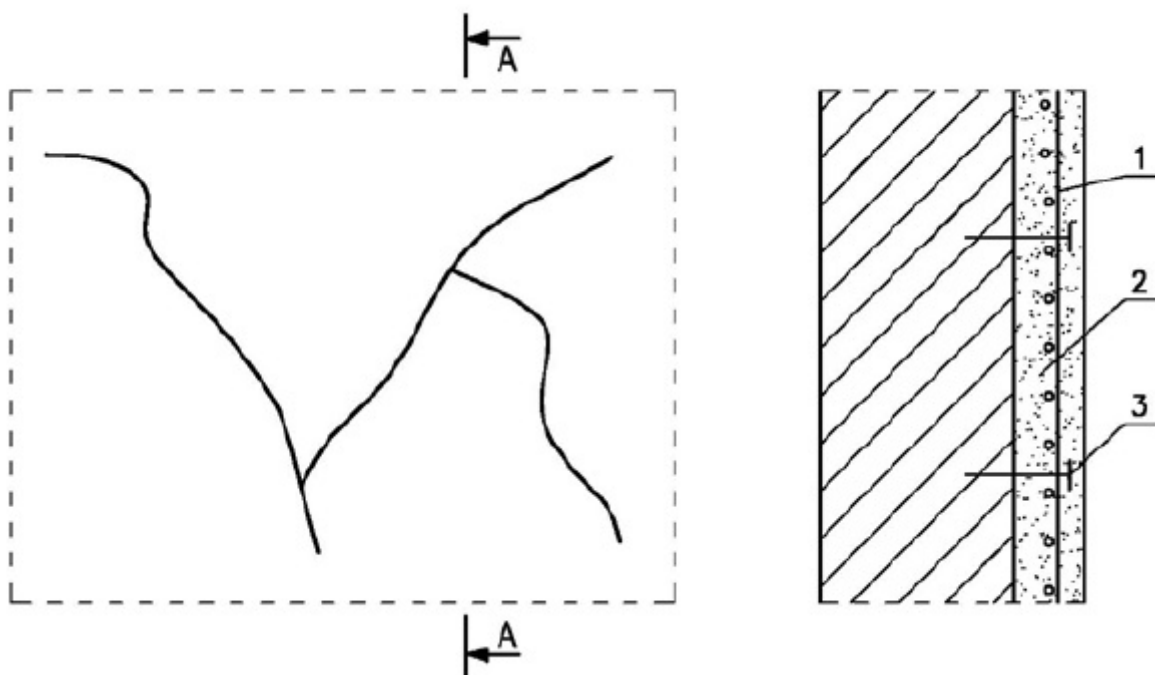
5. Wzmacnianie spękanego muru tynkiem zbrojonym: 1 - siatka zbrojeniowa, 2 - warstwa tynku, 3 - kotwy
