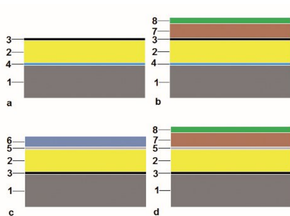
Rys. 4. Schematy stropodachów: 1 - płyta stropodachu, 2 - izolacja cieplna, 3 - izolacja wodochronna, 4 - paroizolacja, 5 - włóknina, 6 - warstwa dociskowa, 7 - ziemia uprawna, 8 - roślinność
