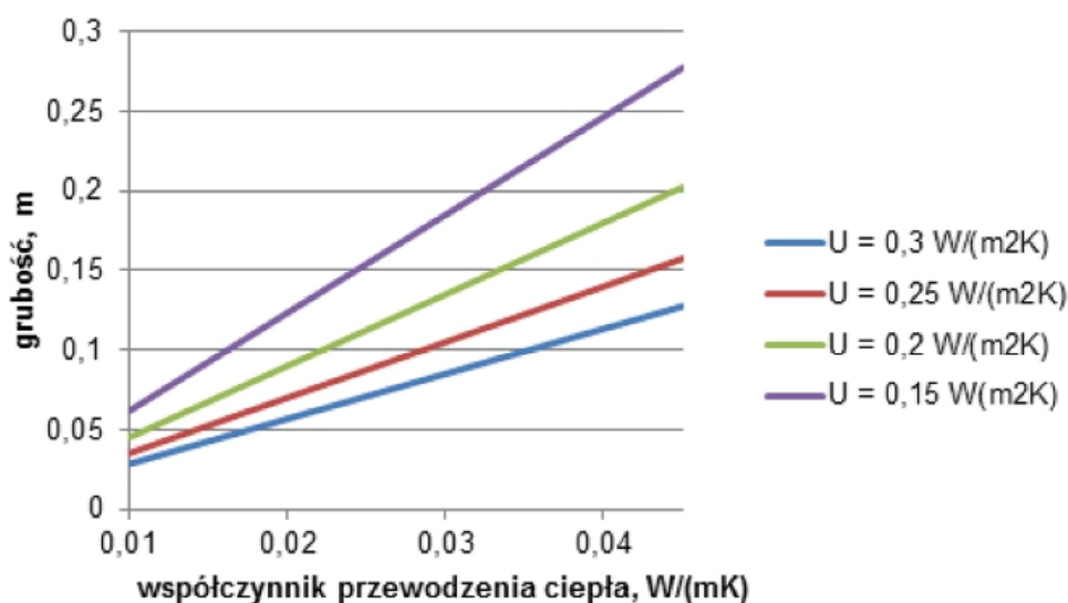
Rys. 7. Grubości izolacji cieplnej, w zależności od jej współczynnika przewodzenia ciepła, przy przyjęciu których uzyskuje się wartość współczynnika przenikania ciepła przegrody od 0,3 do 0,15 W/(m²K). W obliczeniach przyjęto łączny opór cieplny pozostałej części przegrody równy 0,5 m²K/W oraz pominięto wpływ mocowania warstwy izolacji cieplnej
