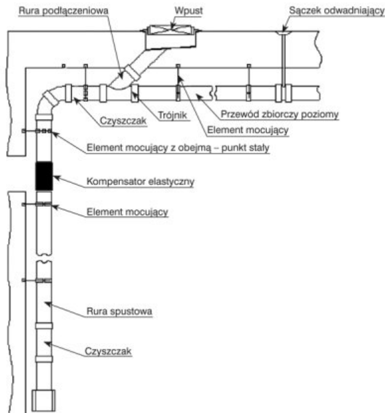
Rys. 1. Standardowe elementy instalacji odprowadzającej wodę z obiektów mostowych
