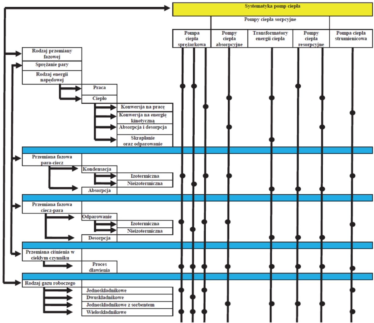
Rys. 2. Systematyka pomp ciepła [1]
